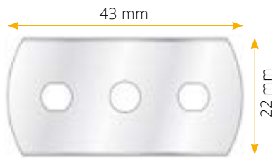
43 x 22 x Kalınlık / Thickness
