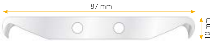
87 x 10 x 0.7 mm
