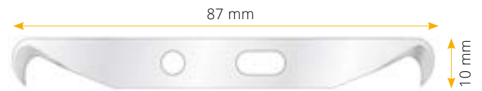
87 x 10 x 0.7 mm
